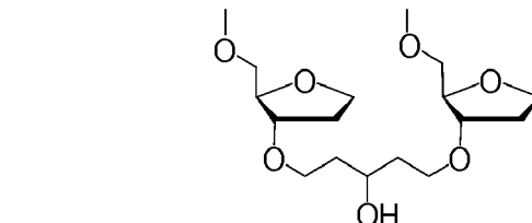
Bis-1,5-O-(3'-thymidyl)-1,3,5-pentanetriol Linker
