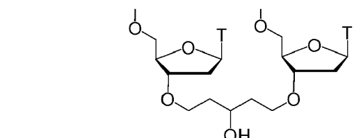
Bis-1,5-O-(3'-thymidyl)-1,3,5-pentanetriol Linker
