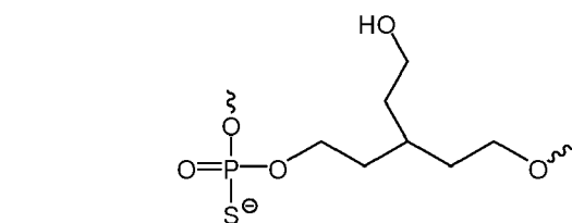
3-(2-Hydroxyethyl)-1,5-pentanediol Linker
