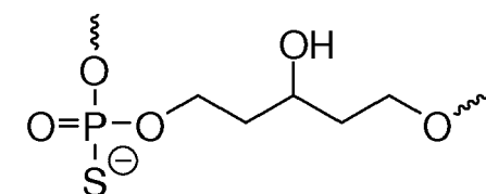
1,3,5-Pentanetriol Linker
