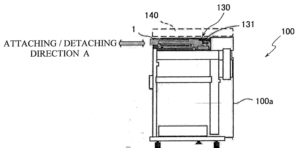
FIG. 1C
