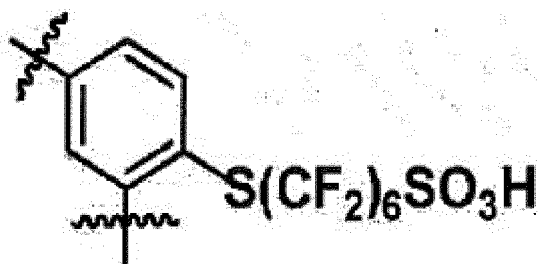
[Formule chimique 1-5]
