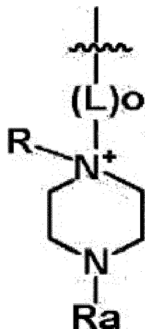
[Formule chimique 1-A]
