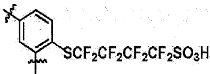
[Formule chimique 1-3]
