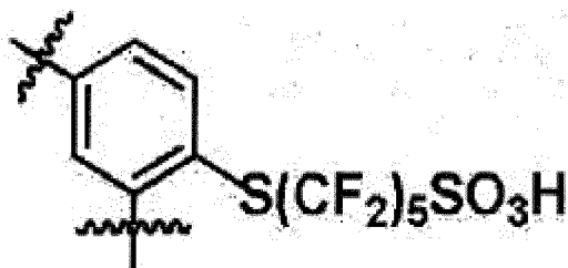
[Formule chimique 1-4]
