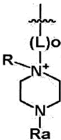
[Formule chimique 1-A]
