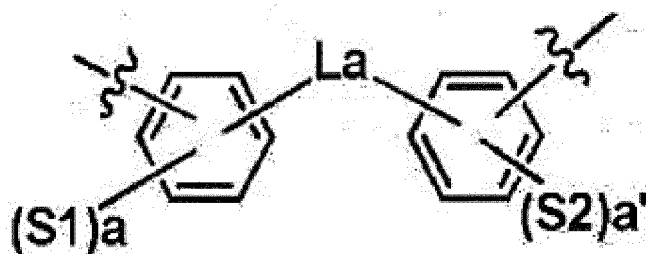
[Formule chimique 2]
