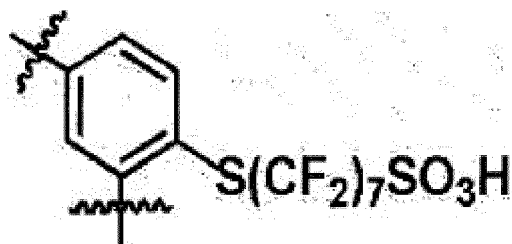
[Formule chimique 1-6]
