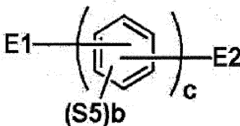
[Formule chimique 3]
