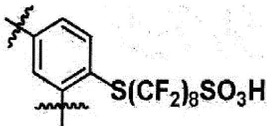
[Formule chimique 1-7]
