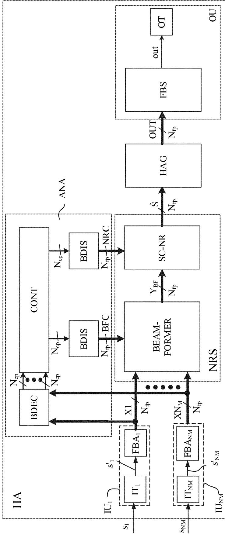
FIG. 1B
