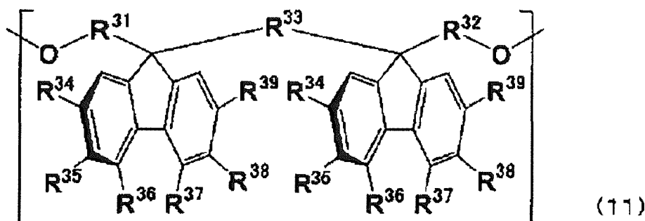
[Chem. 23]
