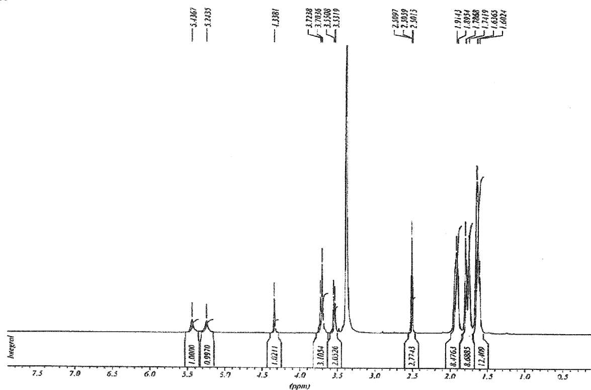
1 H-NMR SPECTRUM OF IN4
