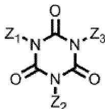
Chemische Formel 2-1
