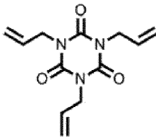
Formule chimique 2-1-1
