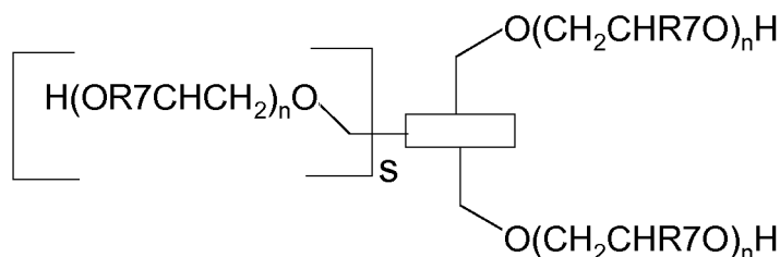
XXXXVI
