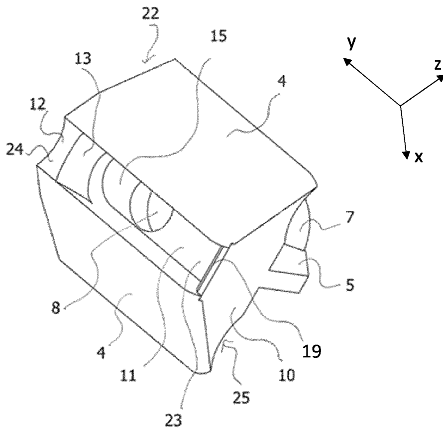
FIG 8F
