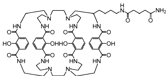
Lumi4®-NH 2
