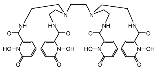
H(2,2)-1,2-HOPO
