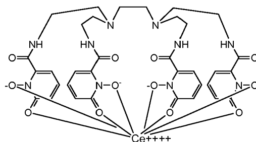
Ce(IV)-H(2,2)-1,2-HOPO
