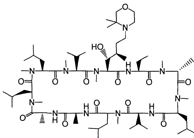
Compound DS
