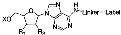
Adenosine N6-linker
