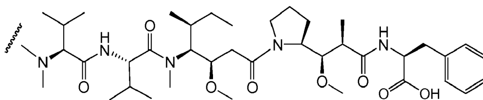
MMAF
