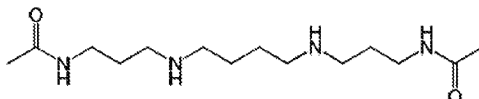
N 1 , N 12 -Diacetylspermine ( N 1 , N 12 -DiAcSPD) N -[3-[4-(3-Acetamidopropylamino)butylamino]propyl]acetamide
