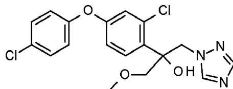
I-27 2-[2-chloro-4-(4-fluorophenoxy)phenyl]-1-methoxy-3-(1,2,4-triazol-1-yl)propan-2-ol:
