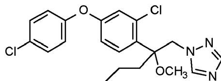
I-23 2-[2-chloro-4-(4-chlorophenoxy)phenyl]-1,1,1-trifluoro-3-(1,2,4-triazol-1-yl)propan-2-ol:
