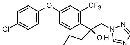
I-29 2-[4-(4-fluorophenoxy)-2-(trifluoromethyl)phenyl]-1-(1,2,4-triazol-1-yl)propan-2-ol:
