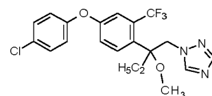
I-14: 2-[4-(4-chlorophenoxy)-2-(trifluoromethyl)phenyl]-1-(1,2,4-triazol-1-yl)pent-3-yn-2-ol
