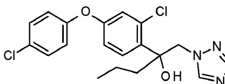
I-31 2-[2-chloro-4-(4-chlorophenoxy)phenyl]-1-(1,2,4-triazol-1-yl)pentan-2-ol:
