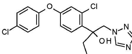
I-31 2-[2-chloro-4-(4-chlorophenoxy)phenyl]-1-(1,2,4-triazol-1-yl)pentan-2-ol:
