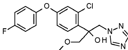
I-28 2-[4-(4-chlorophenoxy)-2-(trifluoromethyl)phenyl]-1-(1,2,4-triazol-1-yl)pentan-2-ol:
