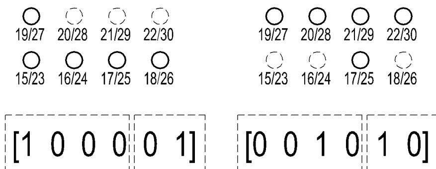
FIG.24
