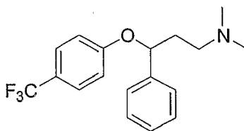
6 N-methylfluoxetine
