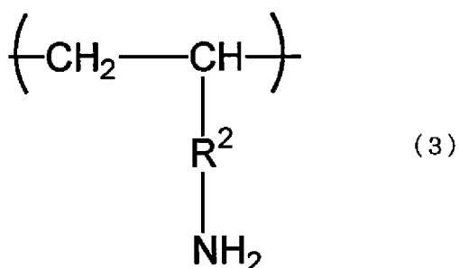
[Chem. 3]
