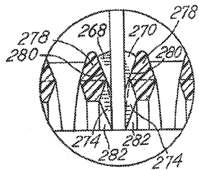
FIG.4IC
