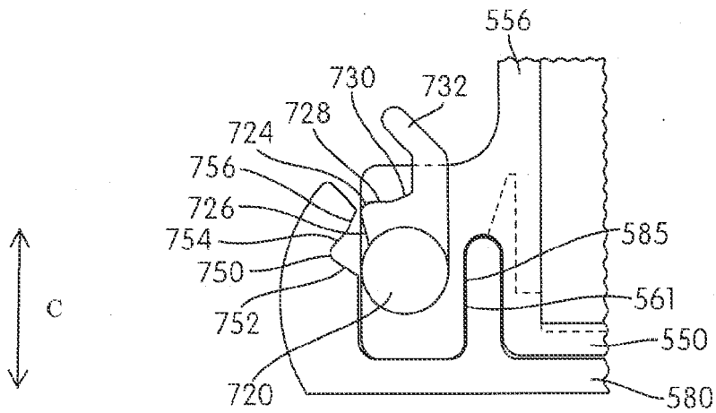
FIG. 87B
