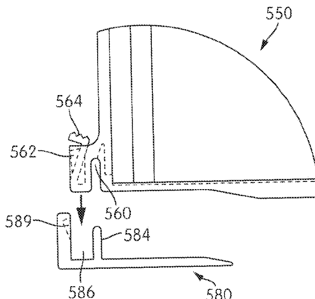
FIG. 68A
