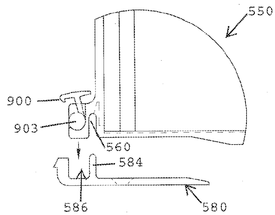
FIG. 89A
