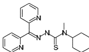
Dp4cycH4mT
