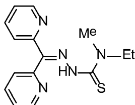
Dp4e4mT
