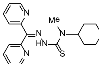
Dp4cycH4mT
