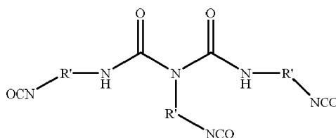
Biuret Trimer
