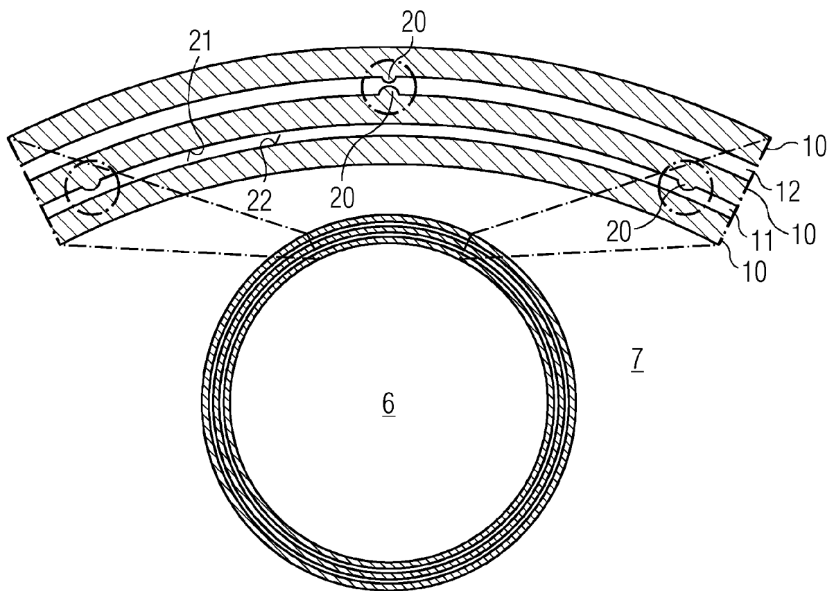
FIG 5 V-V
