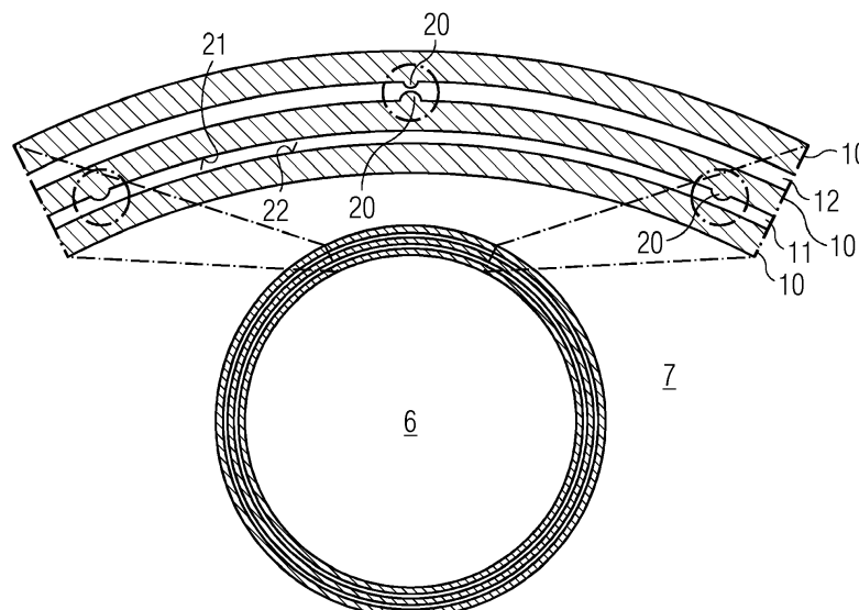
FIG 5 V-V
