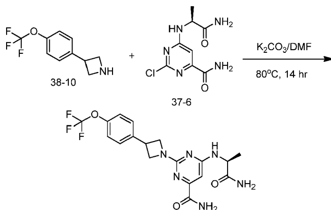
Cpd. No. 101
