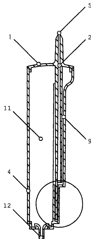
FIG. 5 B-B
