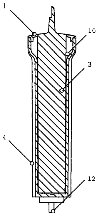
FIG. 4 A-A
