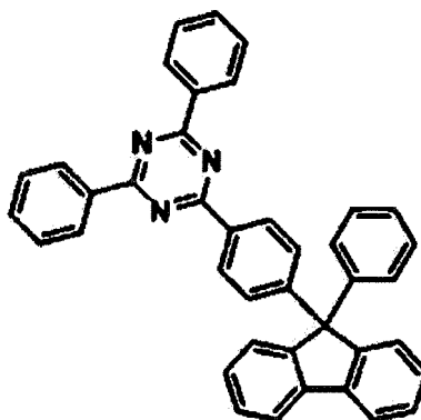
[ET2]
