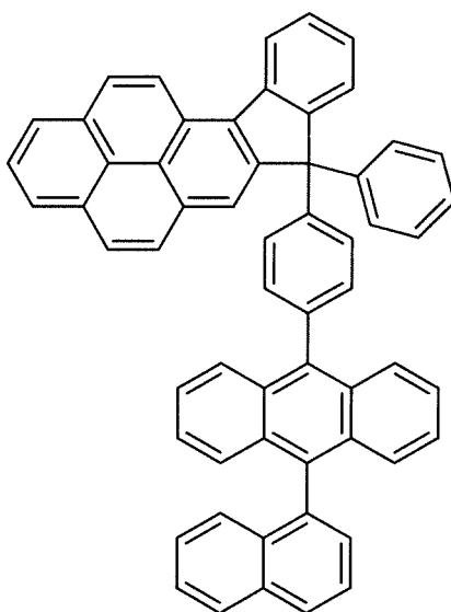
[ET7]
