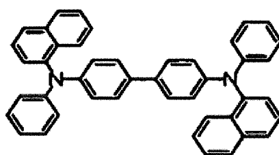
[ HT1 ]
