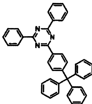
[ET4]
