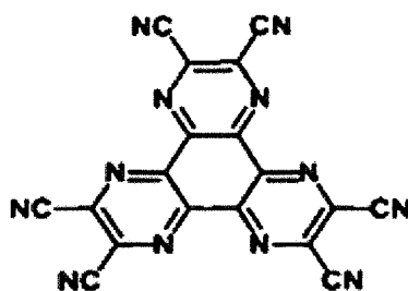
[ HT1 ]
