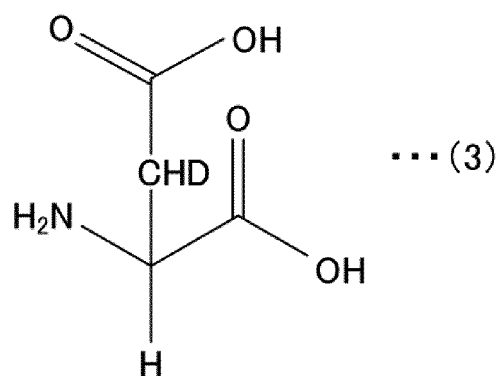
[Chem. 3]
