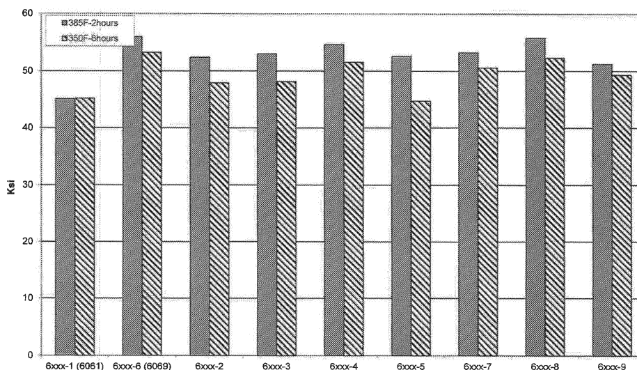
FIG. 1a - Example 1 Alloys - Tensile Yield Strength (ksi)
