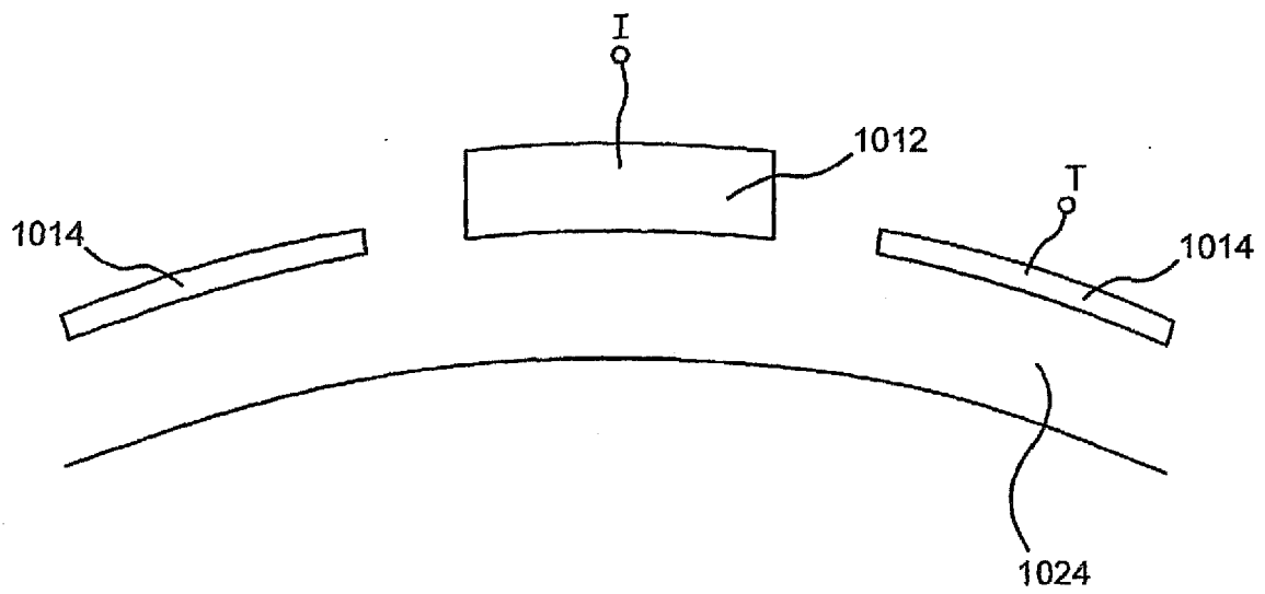
FIG. 10E
