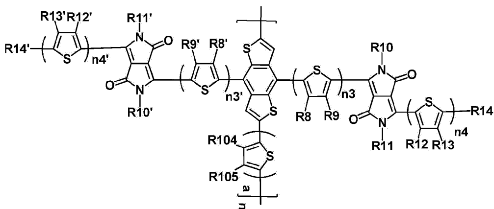
[Chemische Formel 1-3]
