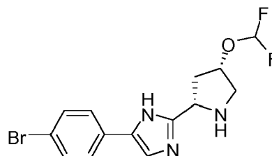
5-(4-Bromo-phenyl)-2-(4-difluoromethoxy- pyrrolidin-2-yl)-1H-imidazole
