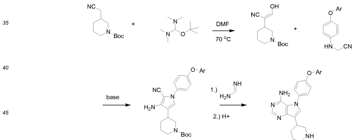
Scheme VI.
