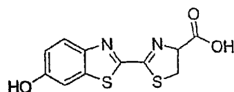
luciferin
