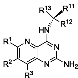
Formula (IVa).
