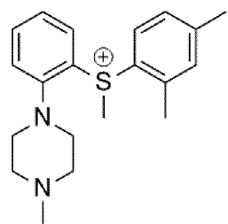
(sulfonium-vortioxetine); Z^-
