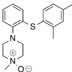
(N-oxide-vortioxetine);
