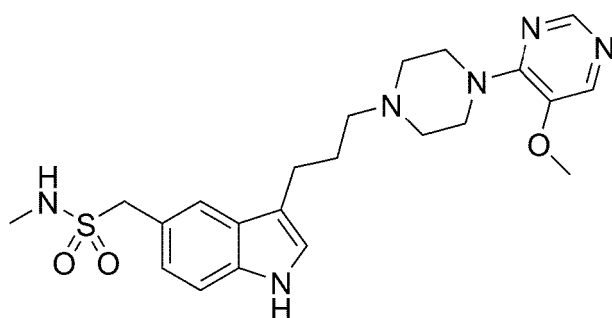
Donitriptan:
