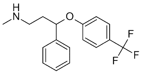
Fluoxetine:
