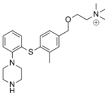
(benzyle-choline-vortioxetine); Z^-
