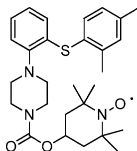
(tempol-carbamate-vortioxetine).
