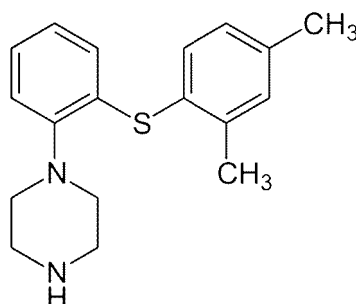
Vortioxetine:
