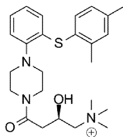
(L-carnitine-vortioxetine); Z^-
