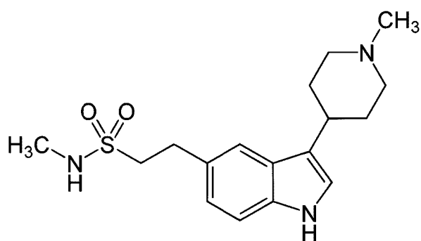
Naratriptan:
