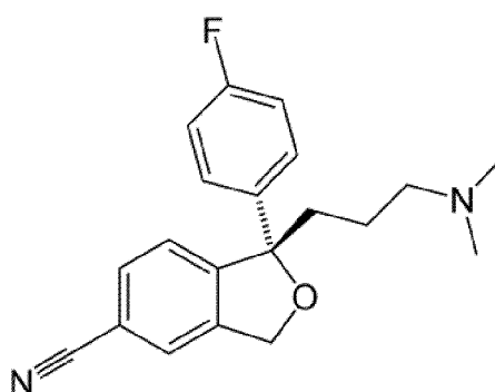
Citalopram:
