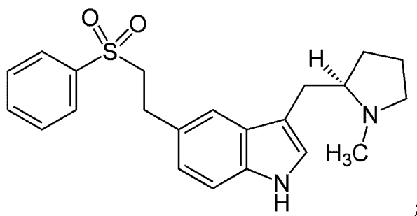
Eletriptan:
