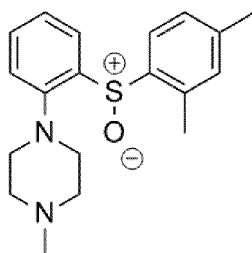
(sulfoxide-vortioxetine);
