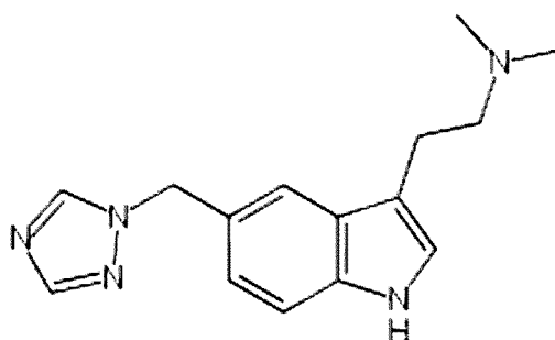
Rizatriptan:
