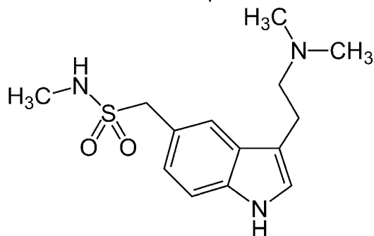
Sumatriptan:
