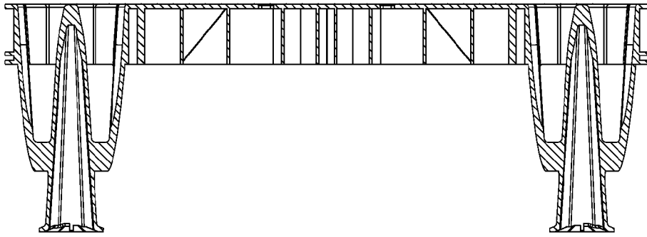
Fig. 80 Section A-A
