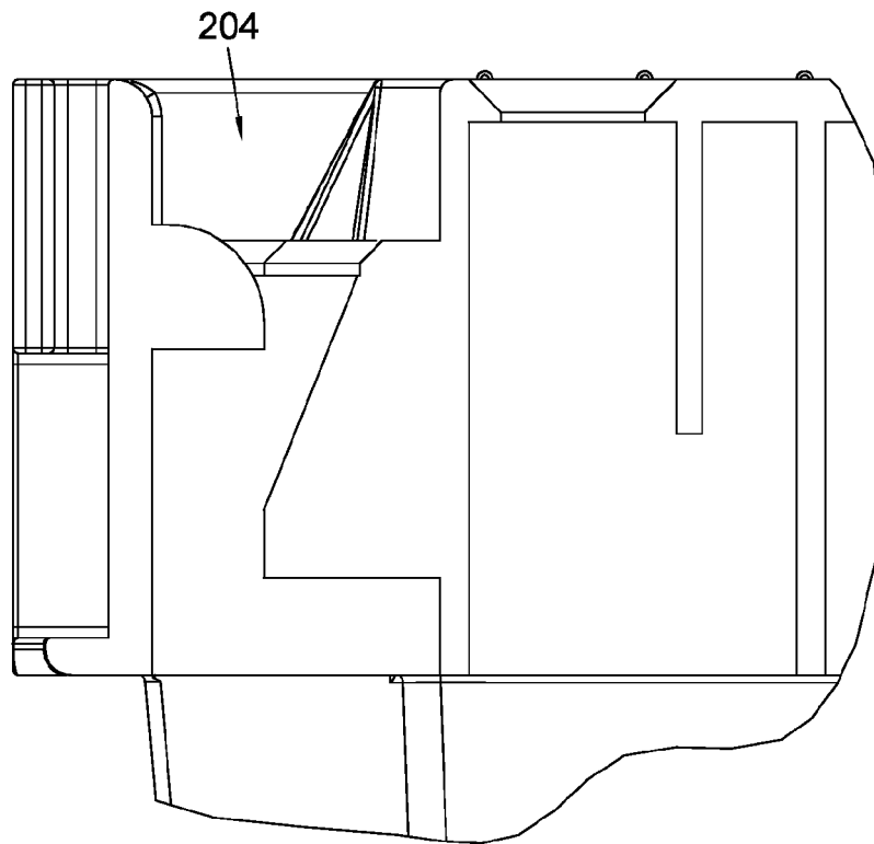
Fig. 74 SECTION D-D
