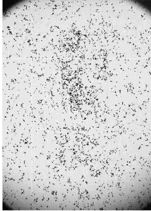
CRISPR-MOSPD2
