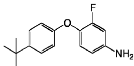
4-(4-(tert-butyl)phenoxy)-3-fluoroaniline,
