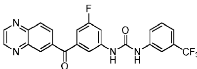
1-(3-fluoro-5-(quinoxaline-6-carbonyl)phenyl)-3-(3-(trifluoromethyl)phenyl)urea
