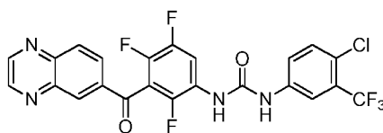
1-(4-chloro-3-(trifluoromethyl)phenyl)-3-(2,4,5-trifluoro-3-(quinoxaline-6-carbonyl)phenyl)urea
