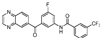
N -(3-fluoro-5-(quinoxaline-6-carbonyl)phenyl)-3-(trifluoromethyl)benzamide
