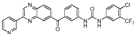
1-(4-chloro-3-(trifluoromethyl)phenyl)-3-(3-(3-(pyridin-3-yl)quinoxaline-6-carbonyl)phenyl)urea
