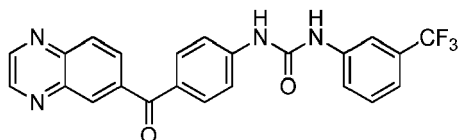
1-(4-(quinoxaline-6-carbonyl)phenyl)-3-(3-(trifluoromethyl)phenyl)urea
