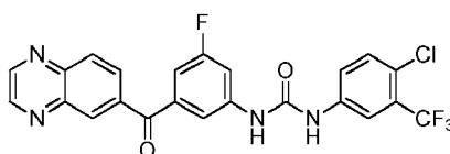
1-(4-chloro-3-(trifluoromethyl)phenyl)-3-(3-fluoro-5-(quinoxaline-6-carbonyl)phenyl)urea
