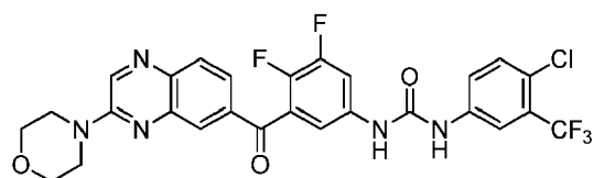
1-(4-chloro-3-(trifluoromethyl)phenyl)-3-(3,4-difluoro-5-(3-morpholinoquinoxaline-6-carbonyl)phenyl)urea
