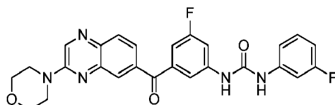
1-(3-fluoro-5-(3-morpholinoquinoxaline-6-carbonyl)phenyl)-3-(3-fluorophenyl)urea
