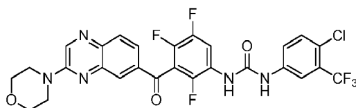
1-(4-chloro-3-(trifluoromethyl)phenyl)-3-(2,4,5-trifluoro-3-(3-morpholinoquinoxaline-6-carbonyl)phenyl)urea
