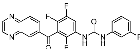
1-(3-fluorophenyl)-3-(2,4,5-trifluoro-3-(quinoxaline-6-carbonyl)phenyl)urea
