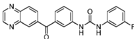
1-(3-fluorophenyl)-3-(3-(quinoxaline-6-carbonyl)phenyl)urea
