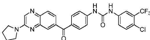
1-(4-chloro-3-(trifluoromethyl)phenyl)-3-(4-(3-(pyrrolidin-1-yl)quinoxaline-6-carbonyl)phenyl)urea
