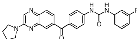
1-(3-fluorophenyl)-3-(4-(3-(pyrrolidin-1-yl)quinoxaline-6-carbonyl)phenyl)urea
