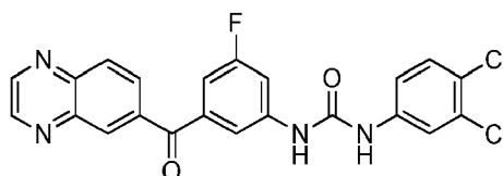
1-(3,4-dichlorophenyl)-3-(3-fluoro-5-(quinoxaline-6-carbonyl)phenyl)urea
