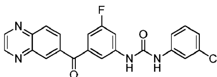
1-(3-chlorophenyl)-3-(3-fluoro-5-(quinoxaline-6-carbonyl)phenyl)urea
