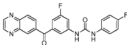
1-(3-fluoro-5-(quinoxaline-6-carbonyl)phenyl)-3-(4-fluorophenyl)urea
