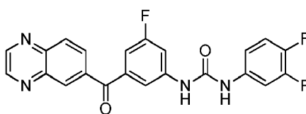
1-(3,4-difluorophenyl)-3-(3-fluoro-5-(quinoxaline-6-carbonyl)phenyl)urea
