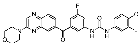
1-(4-chloro-3-fluorophenyl)-3-(3-fluoro-5-(3-morpholinoquinoxaline-6-carbonyl)phenyl)urea
