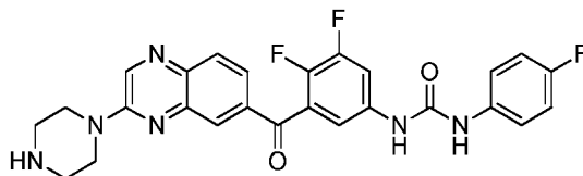
1-(3,4-difluoro-5-(3-(piperazin-1-yl)quinoxaline-6-carbonyl)phenyl)-3-(4-fluorophenyl)urea
