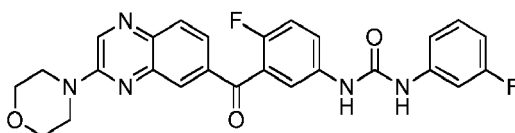
1-(4-fluoro-3-(3-morpholinoquinoxaline-6-carbonyl)phenyl)-3-(3-fluorophenyl)urea
