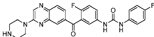
1-(4-fluoro-3-(3-(piperazin-1-yl)quinoxaline-6-carbonyl)phenyl)-3-(4-fluorophenyl)urea
