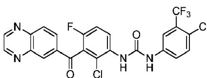
1-(4-chloro-3-(trifluoromethyl)phenyl)-3-(2-chloro-4-fluoro-3-(quinoxaline-6-carbonyl)phenyl)urea
