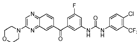
1-(4-chloro-3-(trifluoromethyl)phenyl)-3-(3-fluoro-5-(3-morpholinoquinoxaline-6-carbonyl)phenyl)urea
