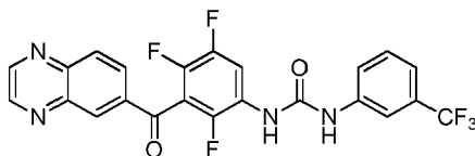
1-(2,4,5-trifluoro-3-(quinoxaline-6-carbonyl)phenyl)-3-(3-(trifluoromethyl)phenyl)urea
