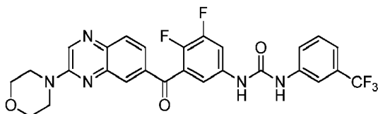
1-(3,4-difluoro-5-(3-morpholinoquinoxaline-6-carbonyl)phenyl)-3-(3-(trifluoromethyl)phenyl)urea
