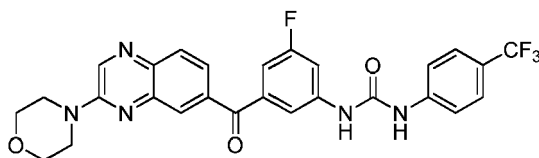
1-(3-fluoro-5-(3-morpholinoquinoxaline-6-carbonyl)phenyl)-3-(4-(trifluoromethyl)phenyl)urea
