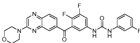
1-(3,4-difluoro-5-(3-morpholinoquinoxaline-6-carbonyl)phenyl)-3-(3-fluorophenyl)urea
