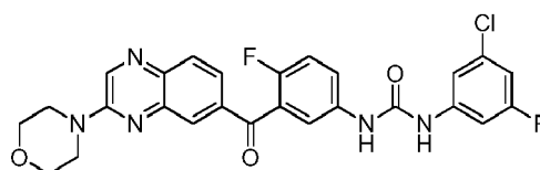
1-(3-chloro-5-fluorophenyl)-3-(4-fluoro-3-(3-morpholinoquinoxaline-6-carbonyl)phenyl)urea
