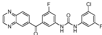
1-(3-chloro-5-fluorophenyl)-3-(3-fluoro-5-(quinoxaline-6-carbonyl)phenyl)urea
