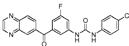
1-(4-chlorophenyl)-3-(3-fluoro-5-(quinoxaline-6-carbonyl)phenyl)urea
