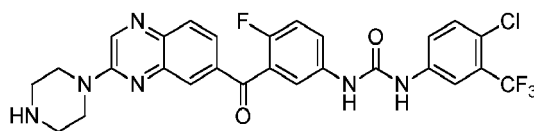
1-(4-chloro-3-(trifluoromethyl)phenyl)-3-(4-fluoro-3-(3-(piperazin-1-yl)quinoxaline-6-carbonyl)phenyl)urea
