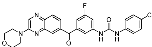
1-(4-chlorophenyl)-3-(3-fluoro-5-(3-morpholinoquinoxaline-6-carbonyl)phenyl)urea
