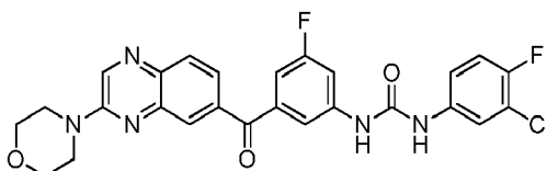
1-(3-chloro-4-fluorophenyl)-3-(3-fluoro-5-(3-morpholinoquinoxaline-6-carbonyl)phenyl)urea
