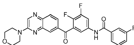
N-(3,4-difluoro-5-(3-morpholinoquinoxaline-6-carbonyl)phenyl)-3-fluorobenzamide
