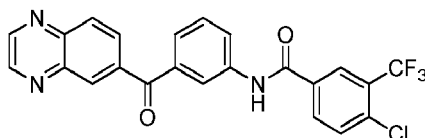
4-chloro-N-(3-(quinoxaline-6-carbonyl)phenyl)-3-(trifluoromethyl)benzamide
