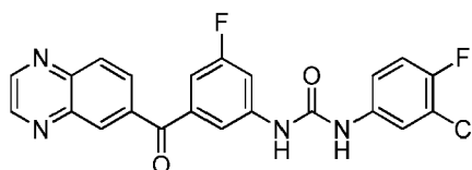
1-(3-chloro-4-fluorophenyl)-3-(3-fluoro-5-(quinoxaline-6-carbonyl)phenyl)urea
