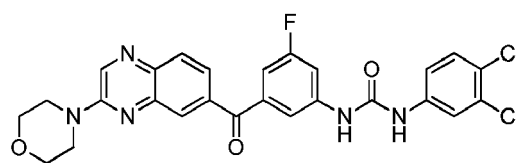
1-(3,4-dichlorophenyl)-3-(3-fluoro-5-(3-morpholinoquinoxaline-6-carbonyl)phenyl)urea
