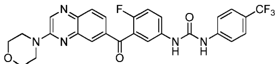
1-(4-fluoro-3-(3-morpholinoquinoxaline-6-carbonyl)phenyl)-3-(4-(trifluoromethyl)phenyl)urea
