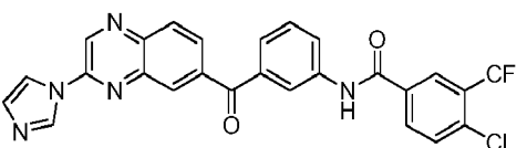
N -(3-(3-(1H-imidazol-1-yl)quinoxaline-6-carbonyl)phenyl)-4-chloro-3-(trifluoromethyl)benzamide
