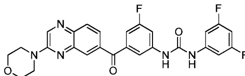
1-(3,5-difluorophenyl)-3-(3-fluoro-5-(3-morpholinoquinoxaline-6-carbonyl)phenyl)urea
