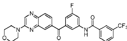
N-(3-fluoro-5-(3-morpholinoquinoxaline-6-carbonyl)phenyl)-3-(trifluoromethyl)benzamide
