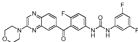
1-(3,5-difluorophenyl)-3-(4-fluoro-3-(3-morpholinoquinoxaline-6-carbonyl)phenyl)urea
