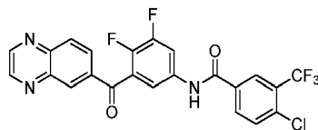
4-chloro-N-(3,4-difluoro-5-(quinoxaline-6-carbonyl)phenyl)-3-(trifluoromethyl)benzamide
