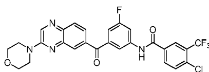
4-chloro- N -(3-fluoro-5-(3-morpholinoquinoxaline-6-carbonyl)phenyl)-3-(trifluoromethyl)benzamide
