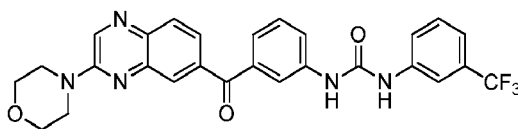
1-(3-(3-morpholinoquinoxaline-6-carbonyl)phenyl)-3-(3-(trifluoromethyl)phenyl)urea
