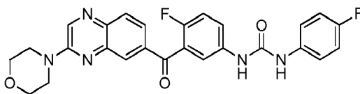
1-(4-fluoro-3-(3-morpholinoquinoxaline-6-carbonyl)phenyl)-3-(4-fluorophenyl)urea
