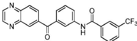
N-(3-(quinoxaline-6-carbonyl)phenyl)-3-(trifluoromethyl)benzamide
