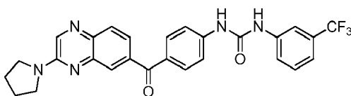
1-(4-(3-(pyrrolidin-1-yl)quinoxaline-6-carbonyl)phenyl)-3-(3-(trifluoromethyl)phenyl)urea
