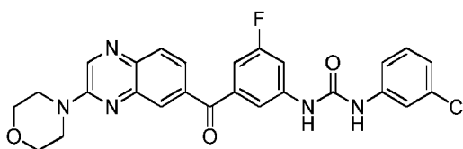
1-(3-chlorophenyl)-3-(3-fluoro-5-(3-morpholinoquinoxaline-6-carbonyl)phenyl)urea
