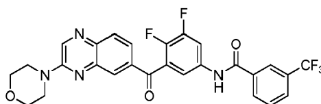
N-(3,4-difluoro-5-(3-morpholinoquinoxaline-6-carbonyl)phenyl)-3-(trifluoromethyl)benzamide
