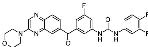
1-(3,4-difluorophenyl)-3-(3-fluoro-5-(3-morpholinoquinoxaline-6-carbonyl)phenyl)urea
