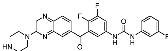
1-(3,4-difluoro-5-(3-(piperazin-1-yl)quinoxaline-6-carbonyl)phenyl)-3-(3-fluorophenyl)urea
