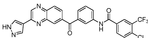
N-(3-(3-(1H-pyrazol-4-yl)quinoxaline-6-carbonyl)phenyl)-4-chloro-3-(trifluoromethyl)benzamide
