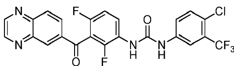
1-(4-chloro-3-(trifluoromethyl)phenyl)-3-(2,4-difluoro-3-(quinoxaline-6-carbonyl)phenyl)urea
