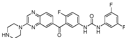
1-(3,5-difluorophenyl)-3-(4-fluoro-3-(3-(piperazin-1-yl)quinoxaline-6-carbonyl)phenyl)urea
