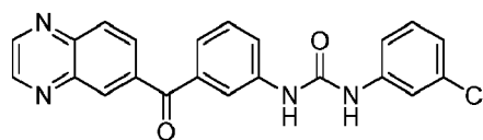
1-(3-chlorophenyl)-3-(3-(quinoxaline-6-carbonyl)phenyl)urea
