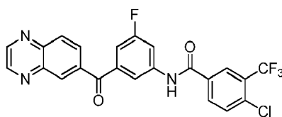
4-chloro- N -(3-fluoro-5-(quinoxaline-6-carbonyl)phenyl)-3-(trifluoromethyl)benzamide
