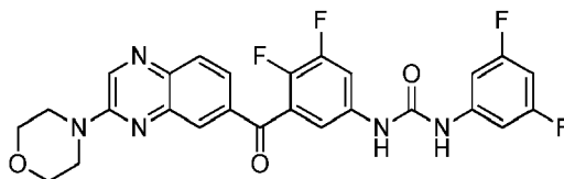
1-(3,4-difluoro-5-(3-morpholinoquinoxaline-6-carbonyl)phenyl)-3-(3,5-difluorophenyl)urea
