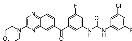
1-(3-chloro-5-fluorophenyl)-3-(3-fluoro-5-(3-morpholinoquinoxaline-6-carbonyl)phenyl)urea
