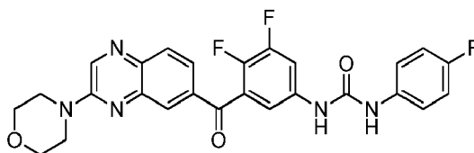
1-(3,4-difluoro-5-(3-morpholinoquinoxaline-6-carbonyl)phenyl)-3-(4-fluorophenyl)urea
