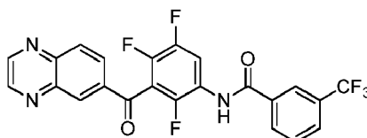
N-(2,4,5-trifluoro-3-(quinoxaline-6-carbonyl)phenyl)-3-(trifluoromethyl)benzamide
