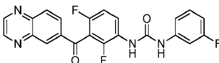
1-(2,4-difluoro-3-(quinoxaline-6-carbonyl)phenyl)-3-(3-fluorophenyl)urea
