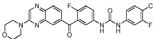
1-(4-chloro-3-fluorophenyl)-3-(4-fluoro-3-(3-morpholinoquinoxaline-6-carbonyl)phenyl)urea
