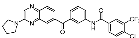
4-chloro- N -(3-(3-(pyrrolidin-1-yl)quinoxaline-6-carbonyl)phenyl)-3-(trifluoromethyl)benzamide
