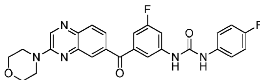
1-(3-fluoro-5-(3-morpholinoquinoxaline-6-carbonyl)phenyl)-3-(4-fluorophenyl)urea
