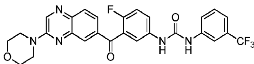
1-(4-fluoro-3-(3-morpholinoquinoxaline-6-carbonyl)phenyl)-3-(3-(trifluoromethyl)phenyl)urea
