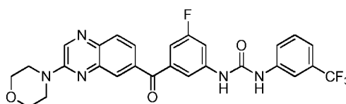
1-(3-fluoro-5-(3-morpholinoquinoxaline-6-carbonyl)phenyl)-3-(3-(trifluoromethyl)phenyl)urea
