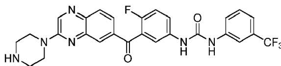
1-(4-fluoro-3-(3-(piperazin-1-yl)quinoxaline-6-carbonyl)phenyl)-3-(3-(trifluoromethyl)phenyl)urea
