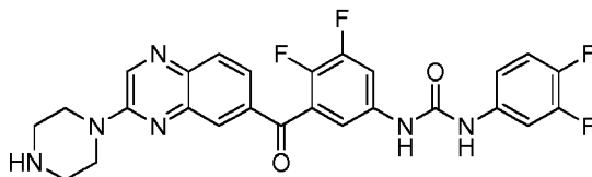
1-(3,4-difluoro-5-(3-(piperazin-1-yl)quinoxaline-6-carbonyl)phenyl)-3-(3,4-difluorophenyl)urea
