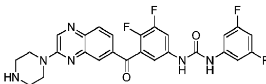
1-(3,4-difluoro-5-(3-(piperazin-1-yl)quinoxaline-6-carbonyl)phenyl)-3-(3,5-difluorophenyl)urea
