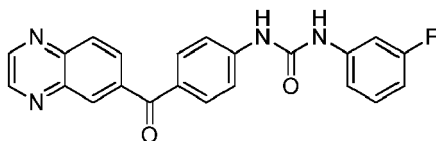
1-(3-fluorophenyl)-3-(4-(quinoxaline-6-carbonyl)phenyl)urea
