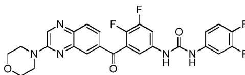
1-(3,4-difluoro-5-(3-morpholinoquinoxaline-6-carbonyl)phenyl)-3-(3,4-difluorophenyl)urea
