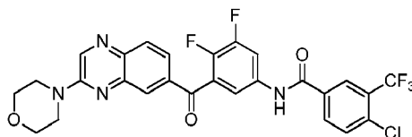
4-chloro- N -(3,4-difluoro-5-(3-morpholinoquinoxaline-6-carbonyl)phenyl)-3-(trifluoromethyl)benzamide
