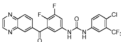
1-(4-chloro-3-(trifluoromethyl)phenyl)-3-(3,4-difluoro-5-(quinoxaline-6-carbonyl)phenyl)urea
