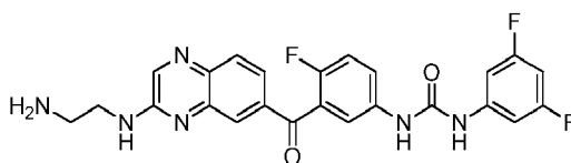
1-(3-(3-((2-aminoethyl)amino)quinoxaline-6-carbonyl)-4-fluorophenyl)-3-(3,5-difluorophenyl)urea
