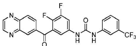
1-(3,4-difluoro-5-(quinoxaline-6-carbonyl)phenyl)-3-(3-(trifluoromethyl)phenyl)urea
