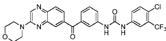
1-(4-chloro-3-(trifluoromethyl)phenyl)-3-(3-(3-morpholinoquinoxaline-6-carbonyl)phenyl)urea
