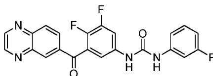
1-(3,4-difluoro-5-(quinoxaline-6-carbonyl)phenyl)-3-(3-fluorophenyl)urea
