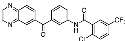
2-chloro- N -(3-(quinoxaline-6-carbonyl)phenyl)-5-(trifluoromethyl)benzamide
