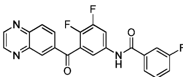
N-(3,4-difluoro-5-(quinoxaline-6-carbonyl)phenyl)-3-fluorobenzamide
