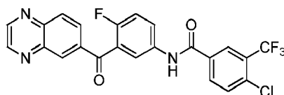
4-chloro-N-(4-fluoro-3-(quinoxaline-6-carbonyl)phenyl)-3-(trifluoromethyl)benzamide
