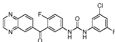
1-(3-chloro-5-fluorophenyl)-3-(4-fluoro-3-(quinoxaline-6-carbonyl)phenyl)urea
