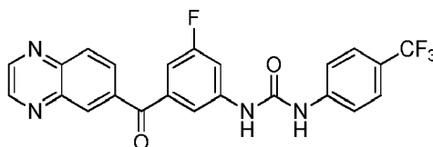
1-(3-fluoro-5-(quinoxaline-6-carbonyl)phenyl)-3-(4-(trifluoromethyl)phenyl)urea
