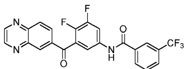
N-(3,4-difluoro-5-(quinoxaline-6-carbonyl)phenyl)-3-(trifluoromethyl)benzamide
