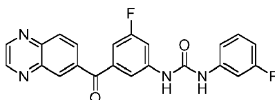
1-(3-fluoro-5-(quinoxaline-6-carbonyl)phenyl)-3-(3-fluorophenyl)urea
