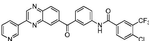
4-chloro- N -(3-(3-(pyridin-3-yl)quinoxaline-6-carbonyl)phenyl)-3-(trifluoromethyl)benzamide
