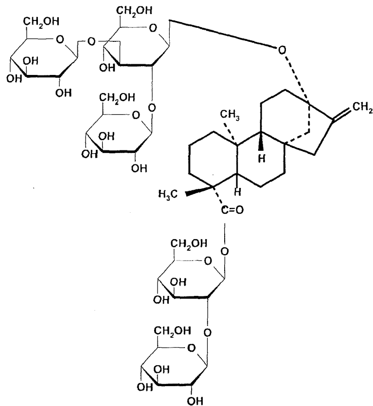
Rebaudioside D
