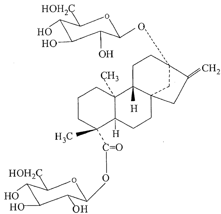
Rubusoside
