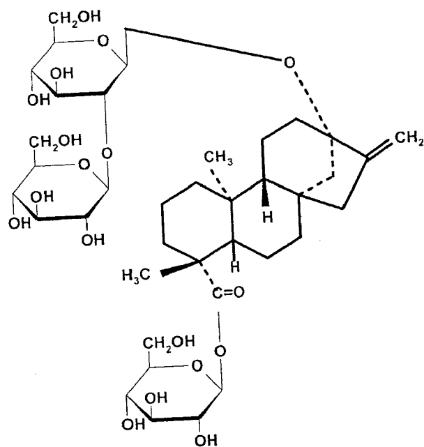
Stevioside
