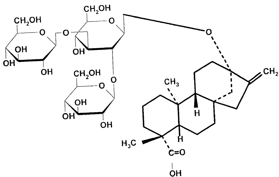
Rebaudioside B
