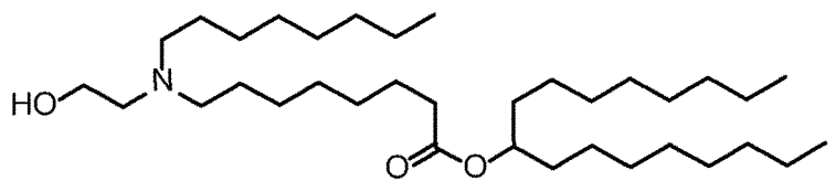
(Composé 4) ,
