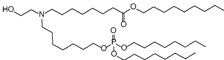
(Composé 131),
