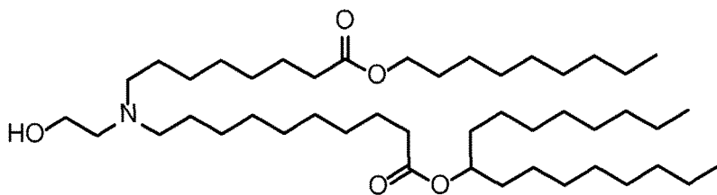
(Composé 23) ,
