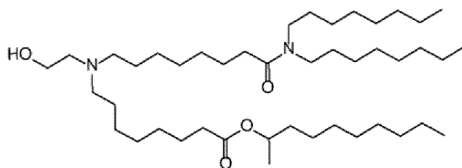
(Verbindung 130),
