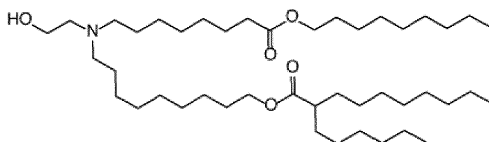
(Verbindung 134),
