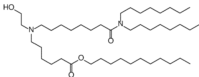
(Composé 129),
