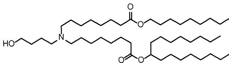
(Composé 20) ,
