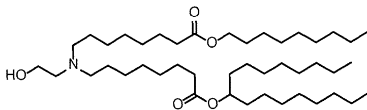
(Composé 18) ,
