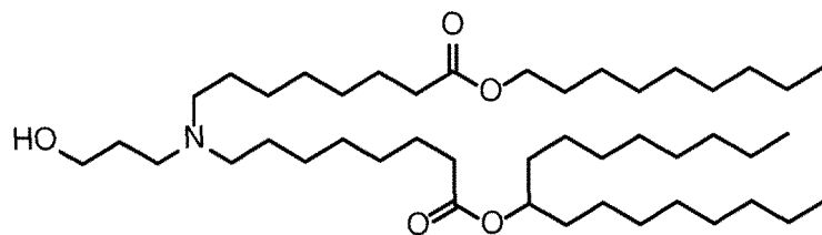
(Composé 19) ,
