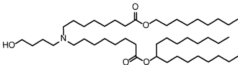
(Verbindung 20),
