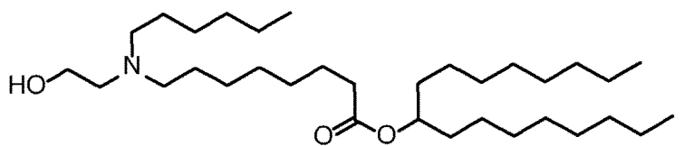
(Composé 5) ,
