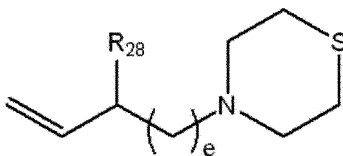
[Formula 28]
