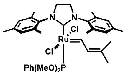
trans-C717
