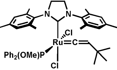
cis -C777v
