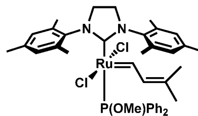
trans -C763
