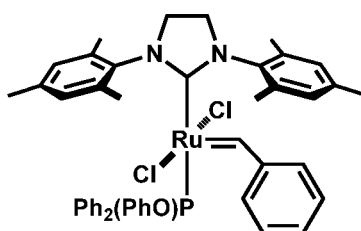
trans -C847
