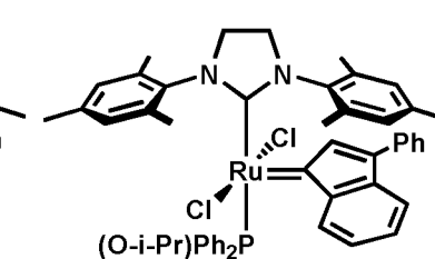
trans -C913
