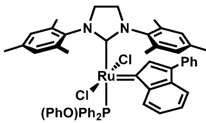
trans -C947
