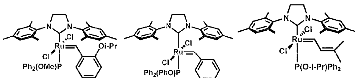
trans -C843
