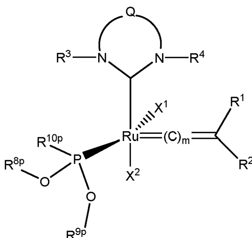
Formula (VIIb)
