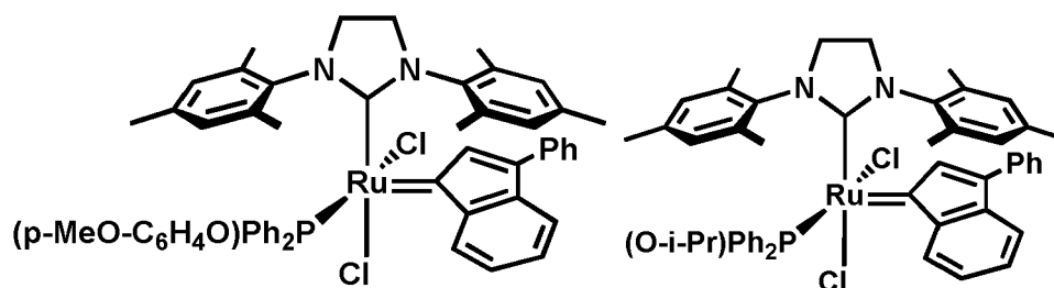
cis -C977
