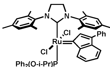
trans -C913
