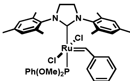
trans -C739
