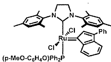
trans -C977
