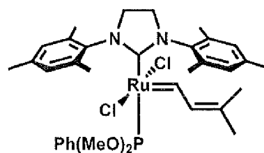
trans -C717
