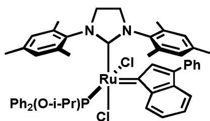
cis -C913
