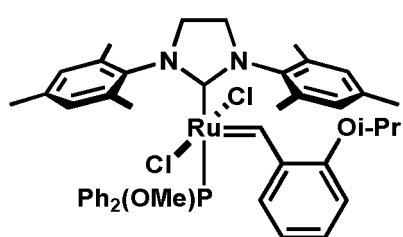
trans -C843
