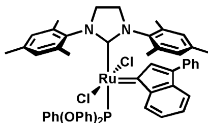
trans-C963
