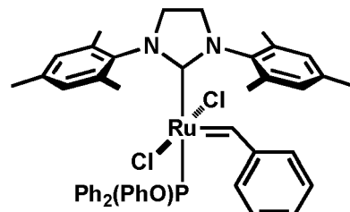
trans -C847
