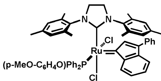
cis -C977
