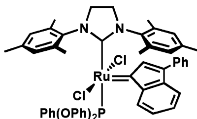
trans-C963
