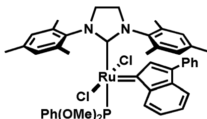
trans -C834
