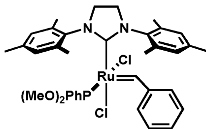
cis-C739
