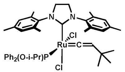
cis -C805v
