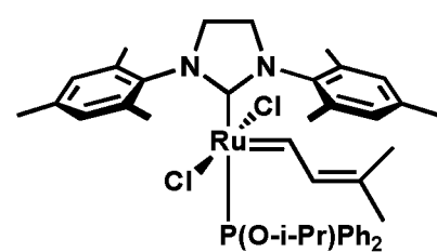
trans -C791
