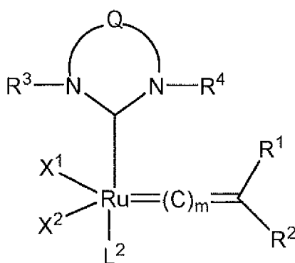
Formel (V)
