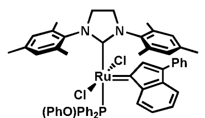
trans -C947
