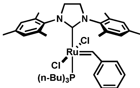
trans-C771
