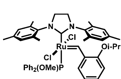
trans -C843
