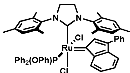
cis-C947
