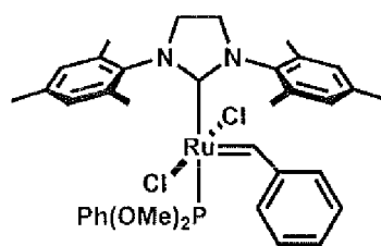
trans -C739
