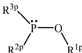
Formule (1)
