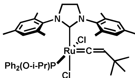
cis-C805v
