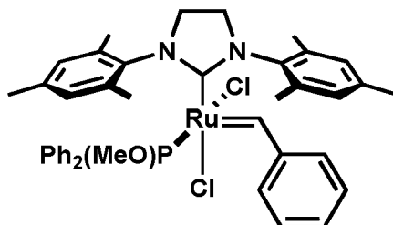
cis -C785
