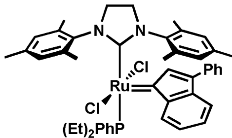
trans-C771
