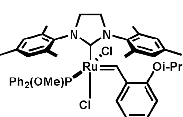
cis -C843
