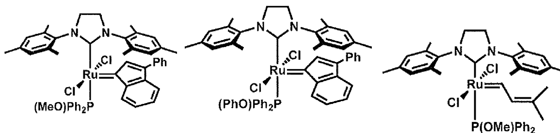
trans -C885
