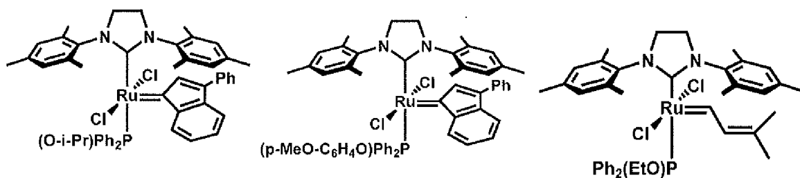
trans -C913
