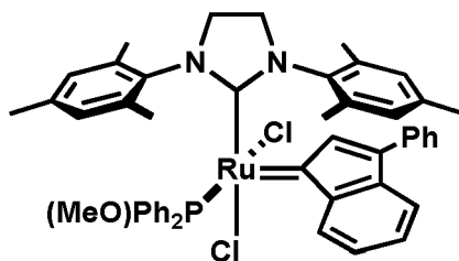
cis-C885
