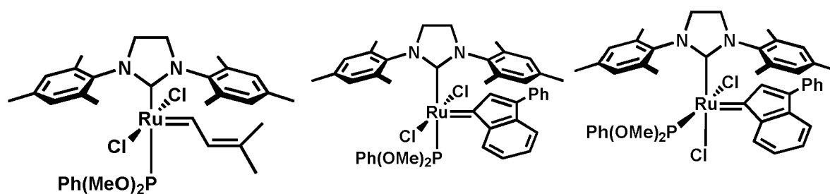
trans -C717
