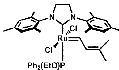
trans -C777
