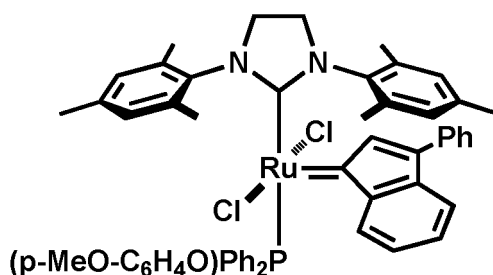
trans -C977
