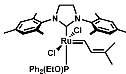
trans -C777
