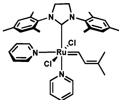
trans-C705
