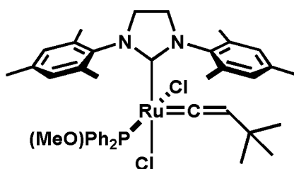
cis-C777v
