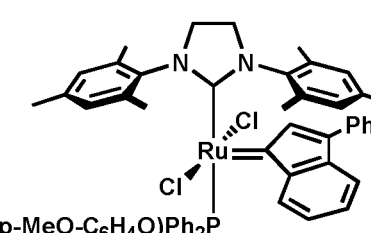
trans -C977
