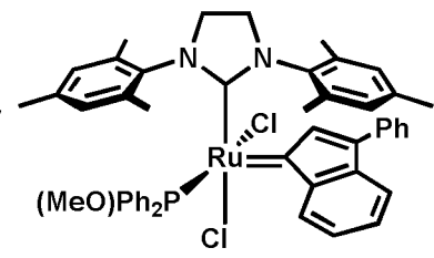
cis -C885
