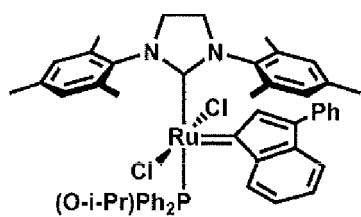
trans -C913
