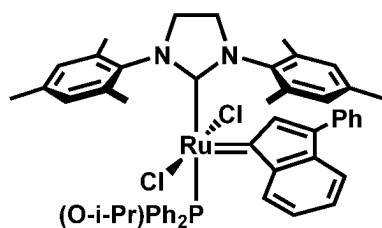
trans -C913
