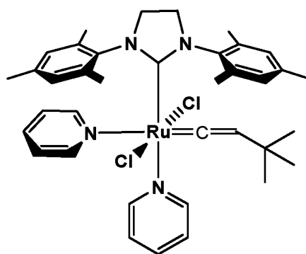
trans-C719v
