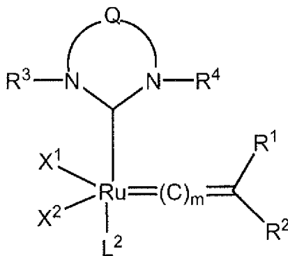
Formel (V)
