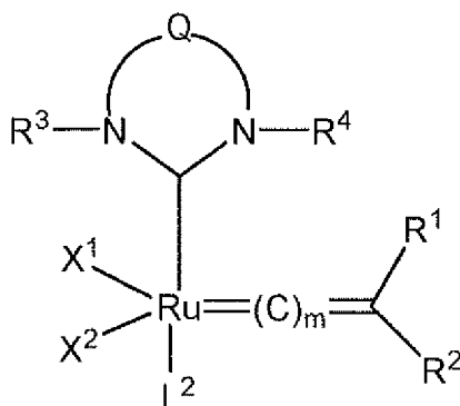
Formule (V)
