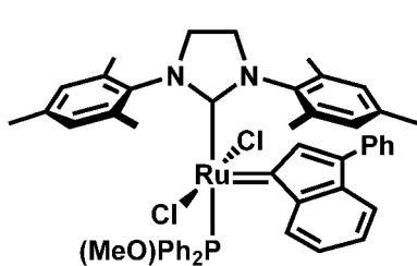
trans -C885
