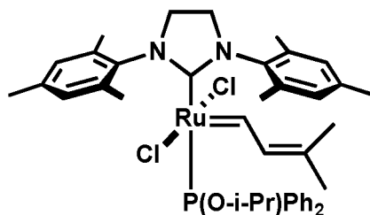
trans-C791
