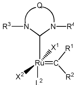
Formula (Va)
