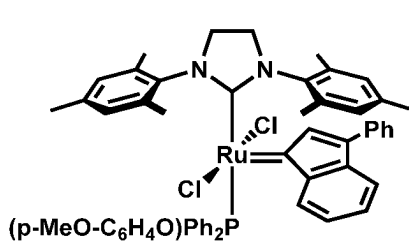
trans -C977
