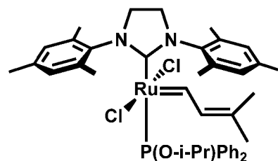
trans -C791
