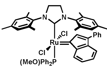
trans -C885
