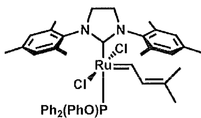
trans -C825
