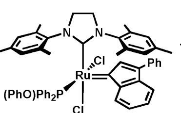
cis -C947
