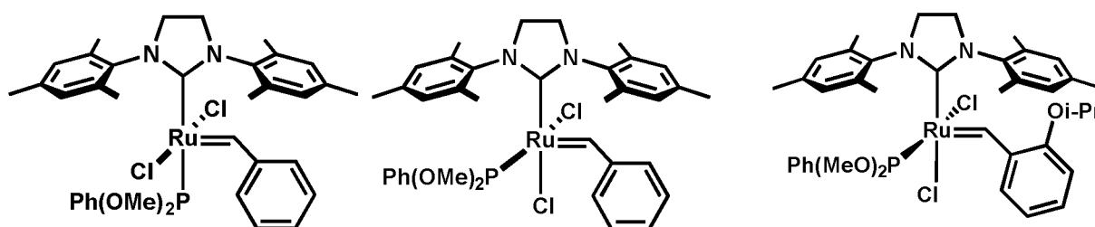
trans -C739
