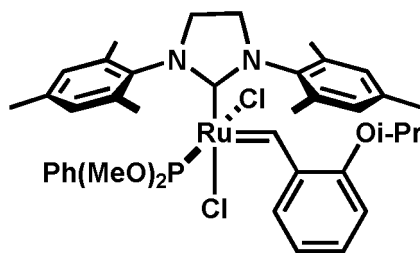
cis-C797
