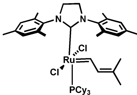
trans-C827
