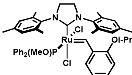
cis-C843
