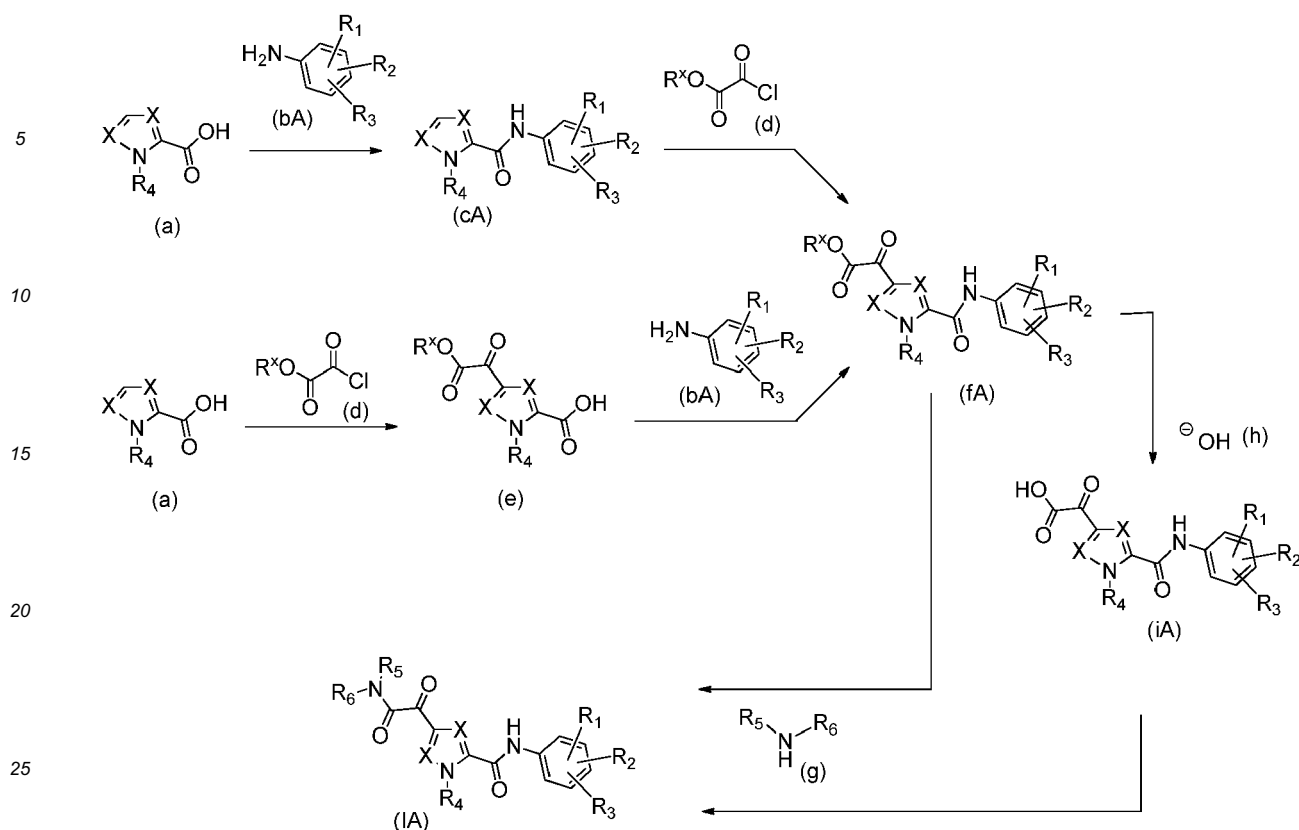
Scheme 1A
