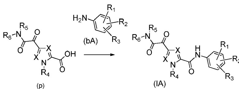
Scheme 2A
