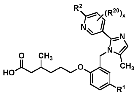
(Ib);
