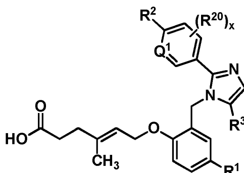
(II); or
