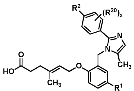
(IIa); or
