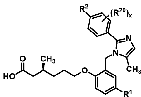
(Iaa');
