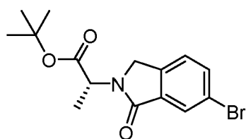
tert-butyl (R)-2-(6-bromo-1-oxisoindolin-2-yl)propanoate
