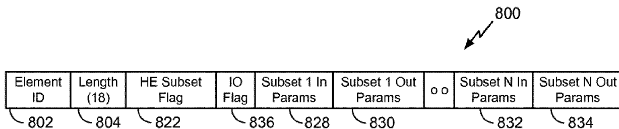
FIG. 8
