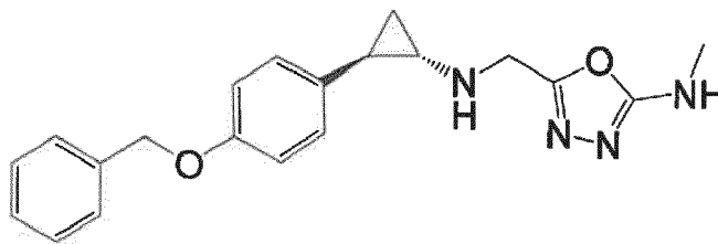
Example 18: N-(5-((((trans)-2-(4-(benzyloxy)phenyl)cyclopropyl)amino)methyl)-1,3,4-oxadiazol-2-yl)acetamide
