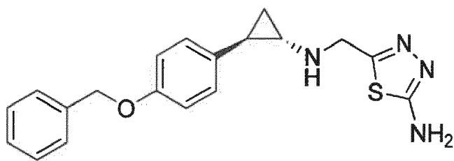
Example 22 : 2-((((trans)-2-(4-(benzyloxy)phenyl)cyclopropyl)amino)methyl)thiazol-5-amine
