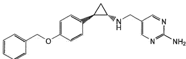
5-((((trans)-2-(4-(benzyloxy)phenyl)cyclopropyl)amino)methyl)pyrimidin-2-amine
