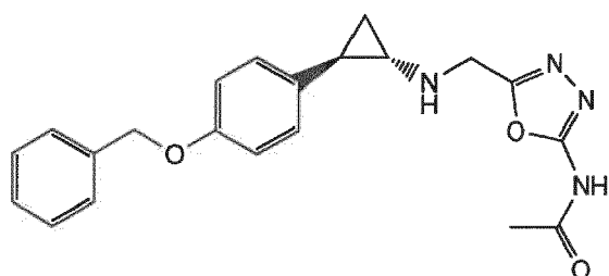
N-(5-((((trans)-2-(4-(benzyloxy)phenyl)cyclopropyl)amino)methyl)-1,3,4-oxadiazol-2-yl)acetamide
