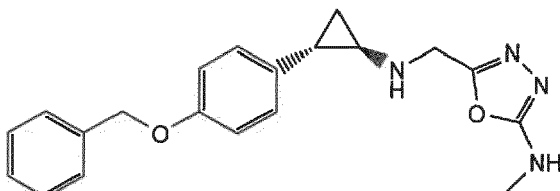
N-(5-((((trans)-2-(4-(benzyloxy)phenyl)cyclopropyl)amino)methyl)-1,3,4-oxadiazol-2-yl)acetamide
