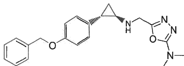
5-((((trans)-2-(4-(benzyloxy)phenyl)cyclopropyl)amino)methyl)-N,N-dimethyl-1,3,4-oxadiazol-2-amine
