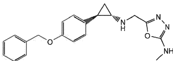
5-((((trans)-2-(4-(benzyloxy)phenyl)cyclopropyl)amino)methyl)-N-methyl-1,3,4-oxadiazol-2-amine
