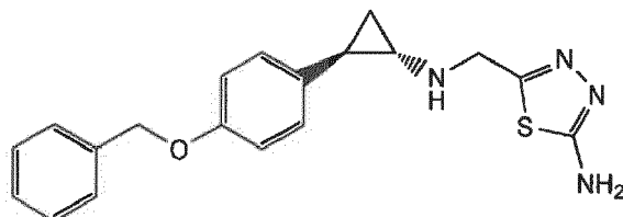
5-((((trans)-2-(4-(benzyloxy)phenyl)cyclopropyl)amino)methyl)-1,3,4-thiadiazol-2-amine
