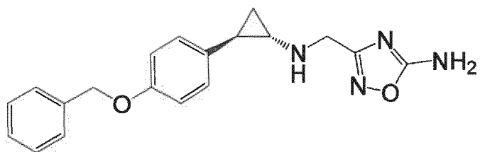
Example 28: 5-((((trans)-2-(4-(benzyloxy)phenyl)cyclopropyl)amino)methyl)-1,2,4-thiadiazol-3-amine
