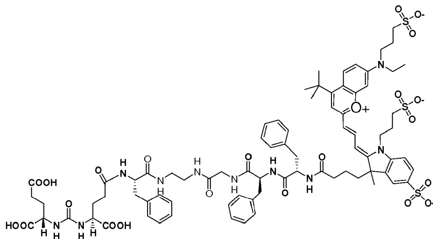
DyLight 800 conjugate
