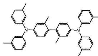
HMTPD
