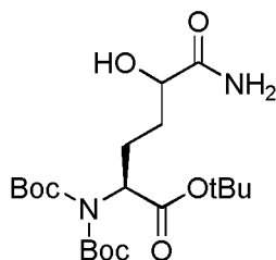
(2S)-tert-butyl 6-amino-2-(bis(tert-butoxycarbonyl)amino)-5-hydroxy-6-oxohexanoate
