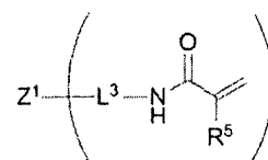
Formula (d)
