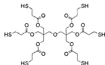
(H-13)
